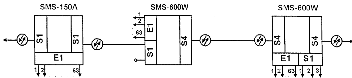
Рисунок А.2 – Система передавання 622 Мбіт/с
