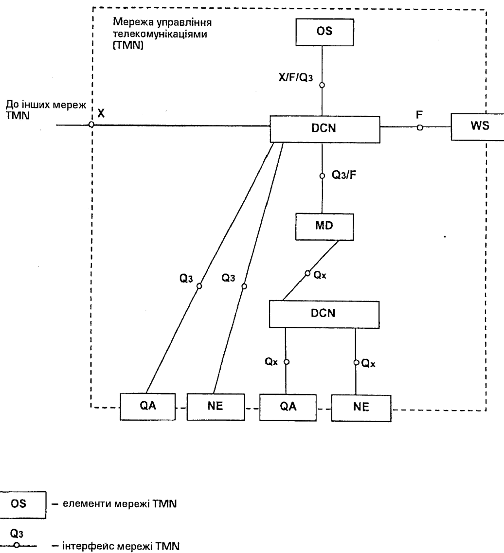
Рисунок Г.2 – Фізична архітектура та інтерфейси мережі управління телекомунікаціями (TMN)
